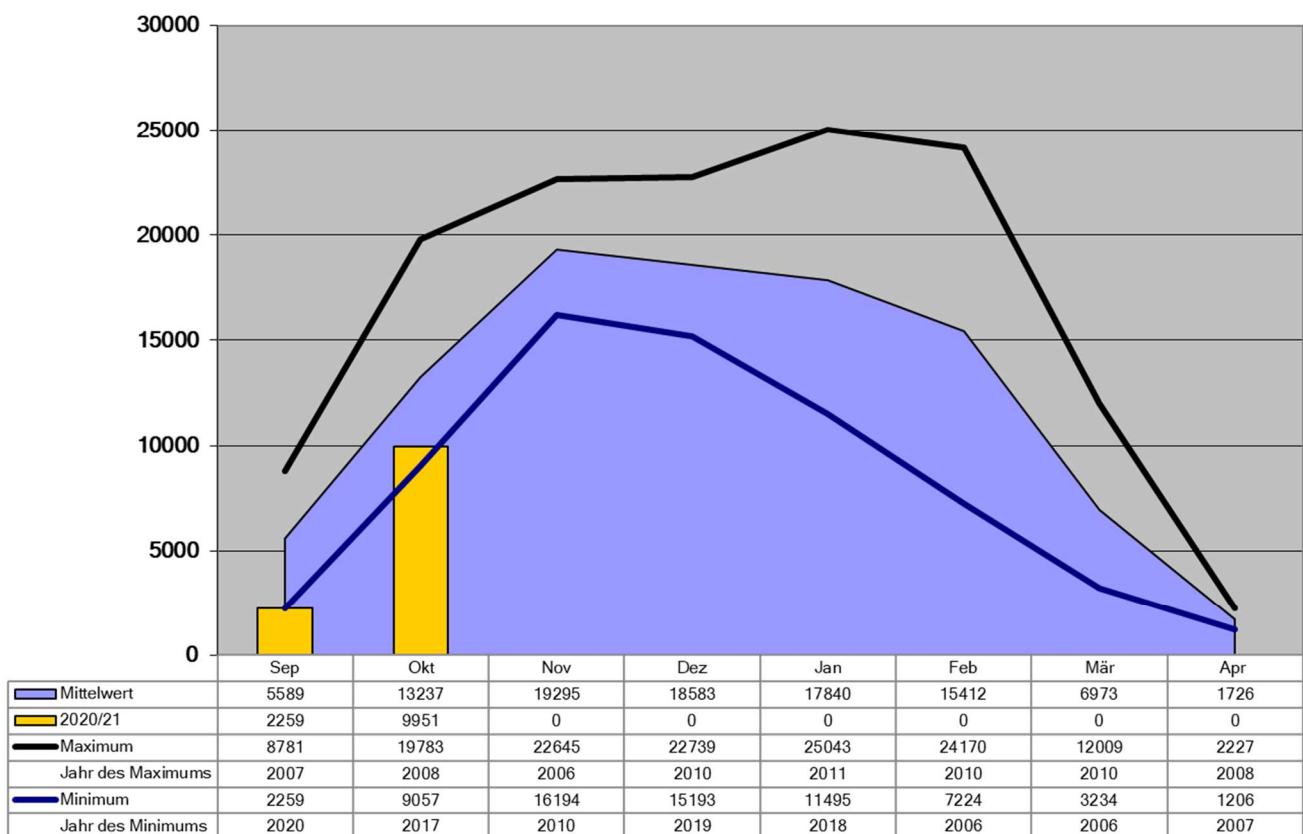
Wasservogelzählung Starnberger See 2003/2004 - 2020/2021
